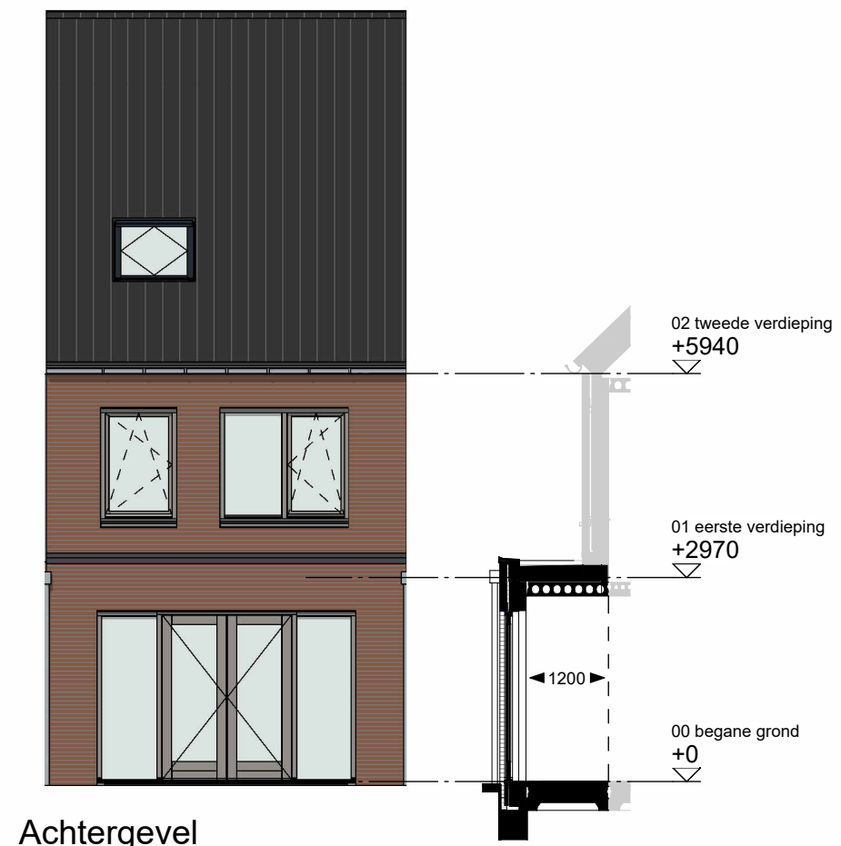
Achtergevel
