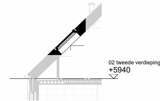
Doorsnede
