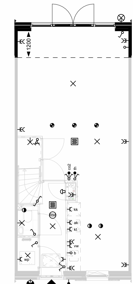
Begane grond
