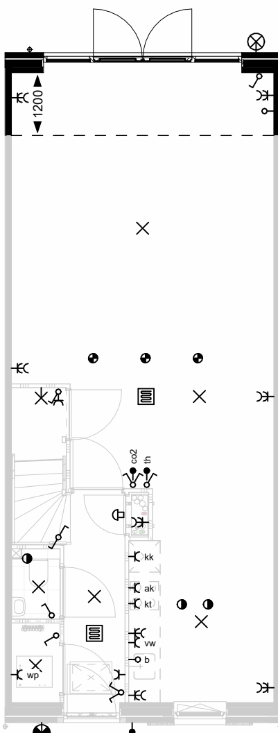
Begane grond
