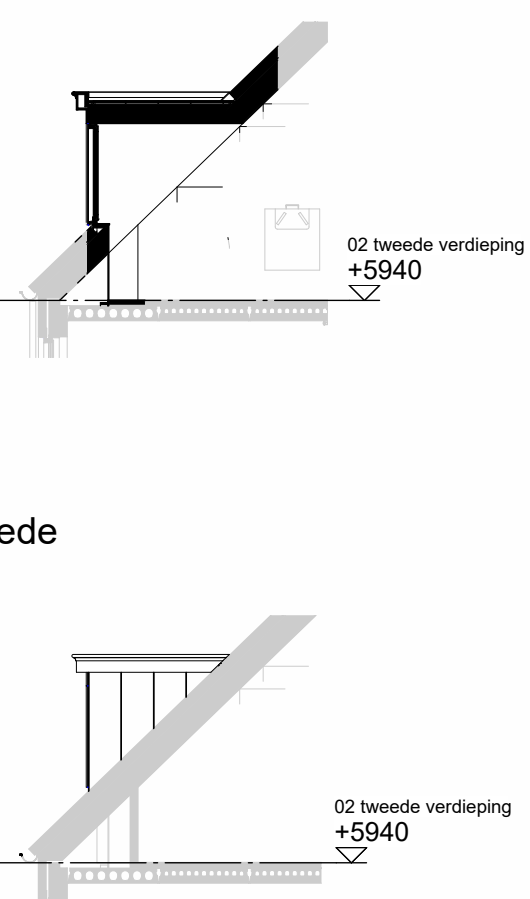
Zijaanzicht
